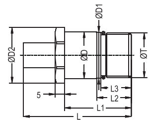
Plug / Nippel
